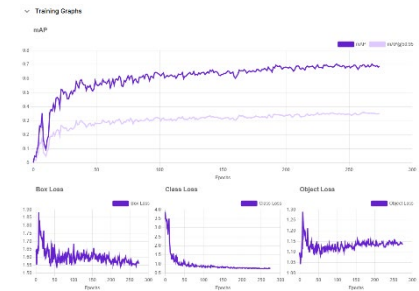
ภาพที่ 7: กราฟแสดงผลลัพธ์การประเมินการดำเนินงานของแพลตฟอร์ม RoboFlow ในการสร้างชุดข้อมูลภาพใหม่
