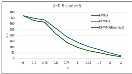
ภาพที่ 10: การเปรียบเทียบค่า ARL ของแผนภูมิควบคุมเมื่อข้อมูลเป็นการแจกแจงลาปลาซ ที่ \lambda = 0.5 และ พารามิเตอร์เท่ากับ 5
