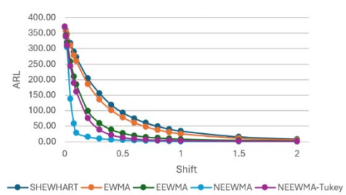
ภาพที่ 4: การเปรียบเทียบค่า ARL ของแผนภูมิ Shewhart EWMA EEWMA NEEWMA และ NEEWMA-Tukey เมื่อกำหนดค่า ARL_0 = 370 ภายใต้การแจกแจงแกมมา
