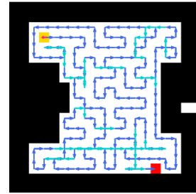
ภาพที่ 8: ผลลัพธ์อัลกอริทึม Random Walk
