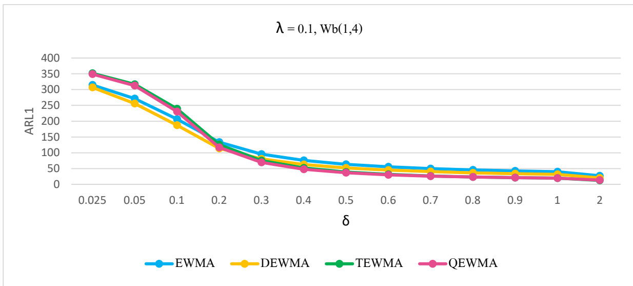
รูปที่: 11 ค่า ARL_1 กรณี \lambda=0.10 ที่มีการแจกแจงไวบูล Wb(1,4) ภายใต้ ARL_0=370
