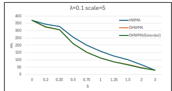
ภาพที่ 8: การเปรียบเทียบค่า ARL ของแผนภูมิควบคุมเมื่อข้อมูลเป็นการแจกแจงลาปลาซ ที่ \lambda = 0.1 และพารามิเตอร์ เท่ากับ 5
