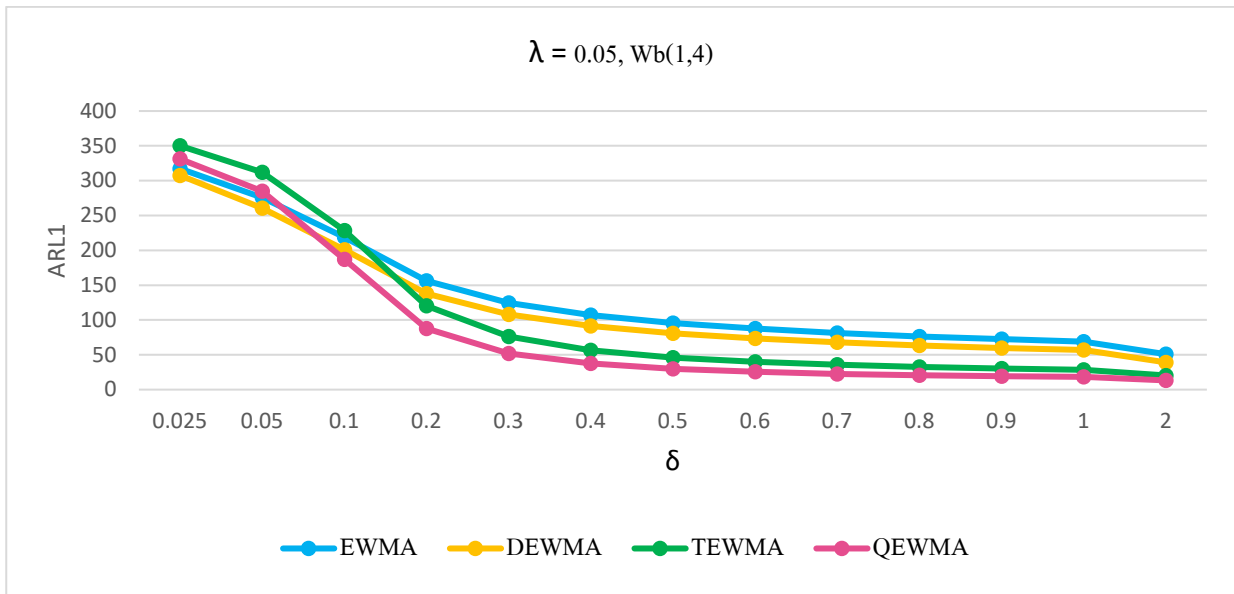
รูปที่: 10 ค่า ARL_1 กรณี \lambda=0.05 ที่มีการแจกแจงไวบูล Wb(1,4) ภายใต้ ARL_0=370
