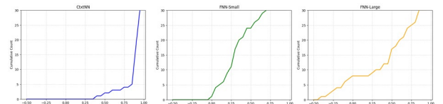
รูปที่ 13: กราฟแสดงการแจกแจง และการแจกแจงสะสมของสัมประสิทธิ์การตัดสินใจของแต่ละตัวแบบ กรณีที่ 3.1
