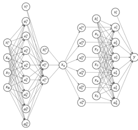
7(a) CtxtNN
