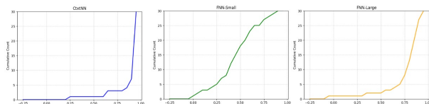
รูปที่ 11: กราฟแสดงการแจกแจง และการแจกแจงสะสมของสัมประสิทธิ์การตัดสินใจของแต่ละตัวแบบ กรณีที่ 2
