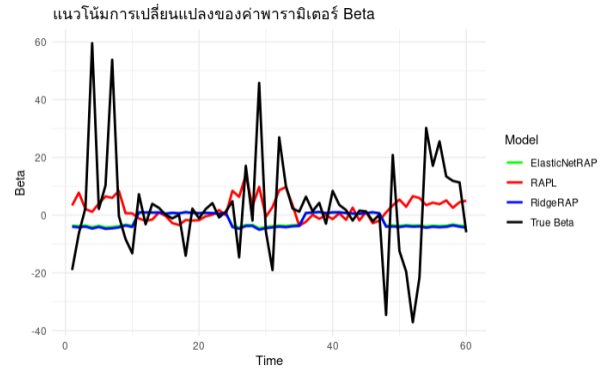
ภาพที่ 2: แนวโน้มการเปลี่ยนแปลงของค่าพารามิเตอร์สัมประสิทธิ์ภายใต้รูปแบบข้อมูลที่มีการเปลี่ยนแปลงสูง
