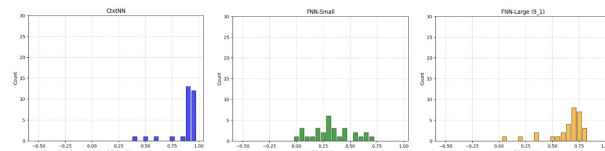
15(a) การแจกแจงของสัมประสิทธิ์การตัดสินใจ
