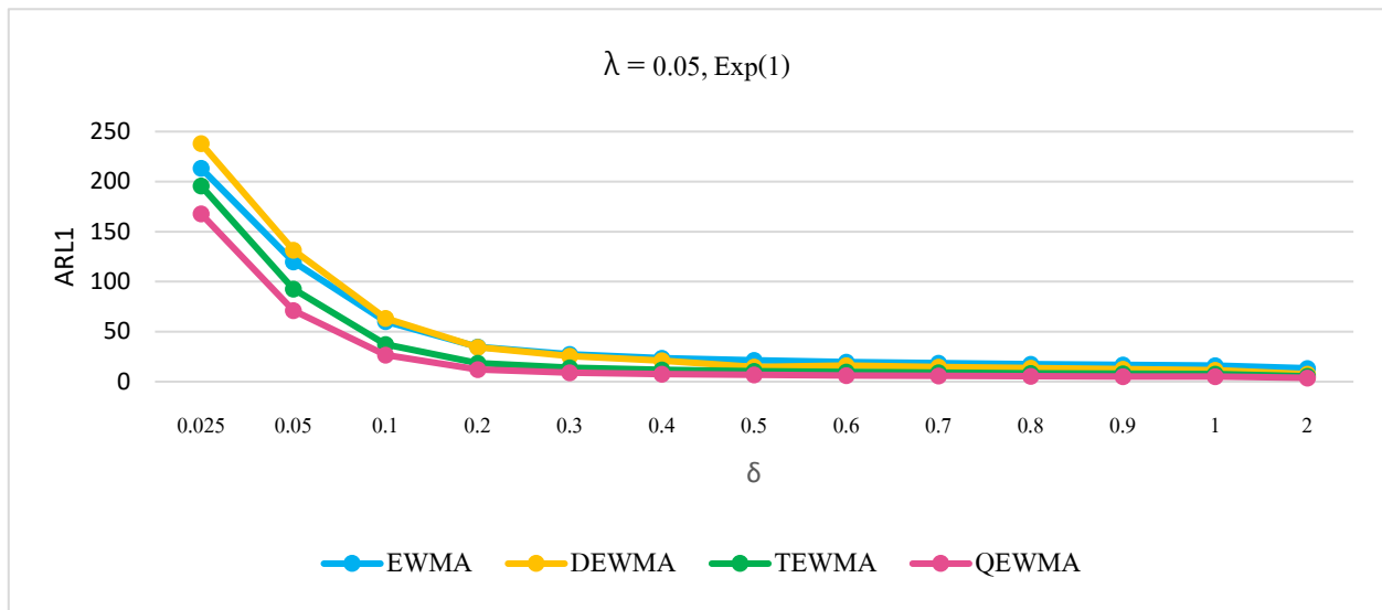
รูปที่: 1 ค่า ARL_1 กรณี \lambda=0.05 ที่มีการแจกแจงแบบเลขชี้กำลัง \text{Exp}(1) ภายใต้ ARL_0=370
