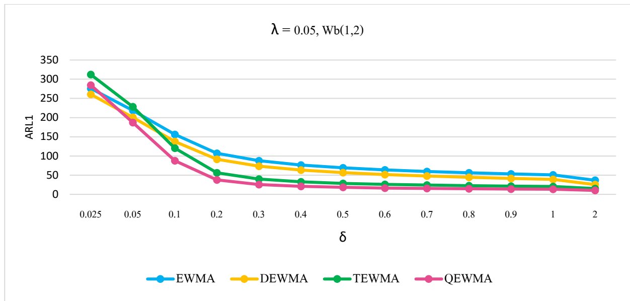
รูปที่: 7 ค่า ARL_1 กรณี \lambda=0.05 ที่มีการแจกแจงไวบูล Wb(1,2) ภายใต้ ARL_0=370
