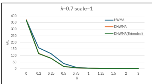
ภาพที่ 11: การเปรียบเทียบค่า ARL ของแผนภูมิควบคุมเมื่อข้อมูลเป็นการแจกแจงลาปลาซ ที่ \lambda = 0.7 และ พารามิเตอร์เท่ากับ 1
