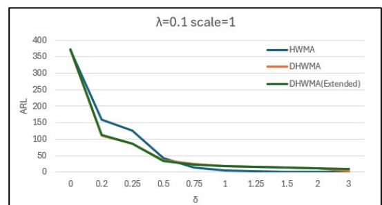
ภาพที่ 7: การเปรียบเทียบค่า ARL ของแผนภูมิควบคุมเมื่อข้อมูลเป็นการแจกแจงลาปลาซ ที่ \lambda = 0.1 และพารามิเตอร์ เท่ากับ 1
