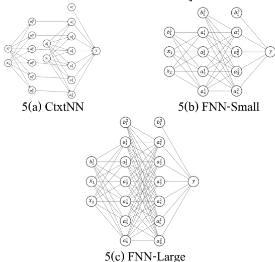
รูปที่ 5: โครงสร้างโครงข่ายประสาทเทียมของตัวแบบ 3 แบบ สำหรับกรณี 1
