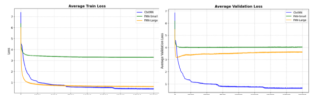
รูปที่ 12: กราฟแสดงการเปรียบเทียบค่าเฉลี่ย MSE (Loss) ในแต่ละ Epoch สำหรับแต่ละตัวแบบ กรณีที่ 3.1
