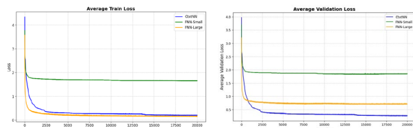
รูปที่ 10: กราฟแสดงการเปรียบเทียบค่าเฉลี่ย MSE (Loss) ในแต่ละ Epoch สำหรับแต่ละตัวแบบ กรณีที่ 2
