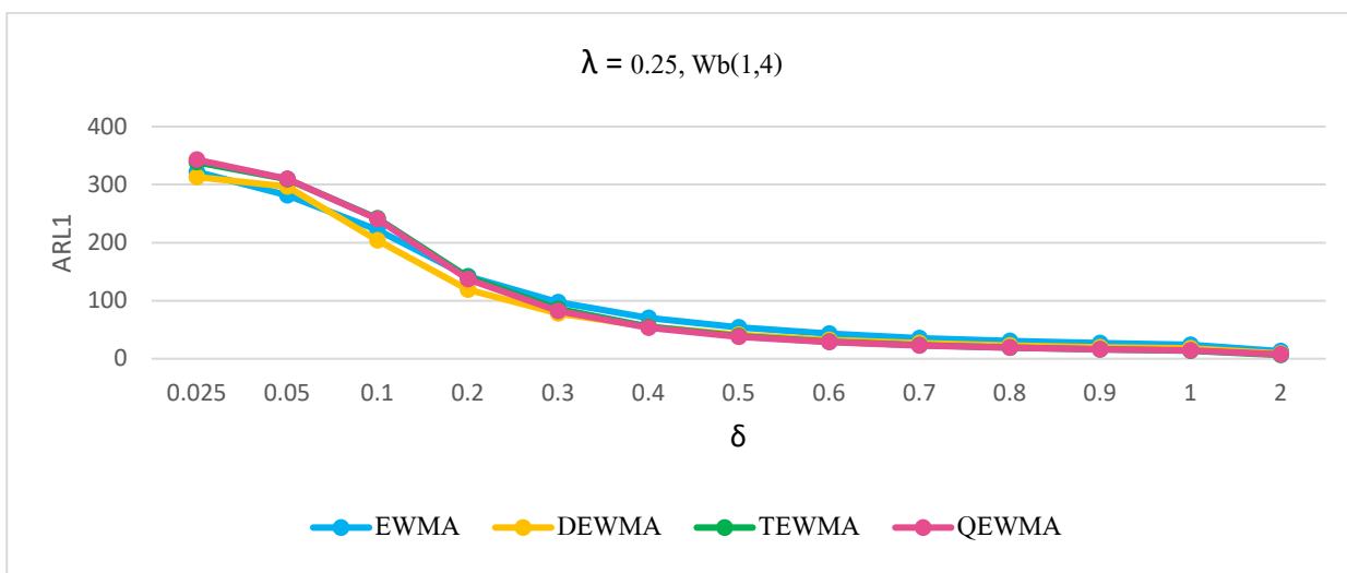
รูปที่: 12 ค่า ARL_1 กรณี \lambda=0.25 ที่มีการแจกแจงไวบูล Wb(1,4) ภายใต้ ARL_0=370
