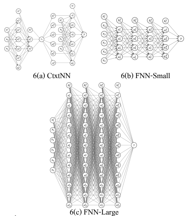
รูปที่ 6: โครงสร้างโครงข่ายประสาทเทียมของตัวแบบ 3 แบบ สำหรับกรณี 2
