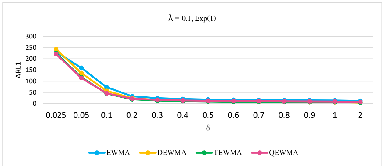
รูปที่: 2 ค่า ARL_1 กรณี \lambda=0.10 ที่มีการแจกแจงแบบเลขชี้กำลัง \text{Exp}(1) ภายใต้ ARL_0=370
