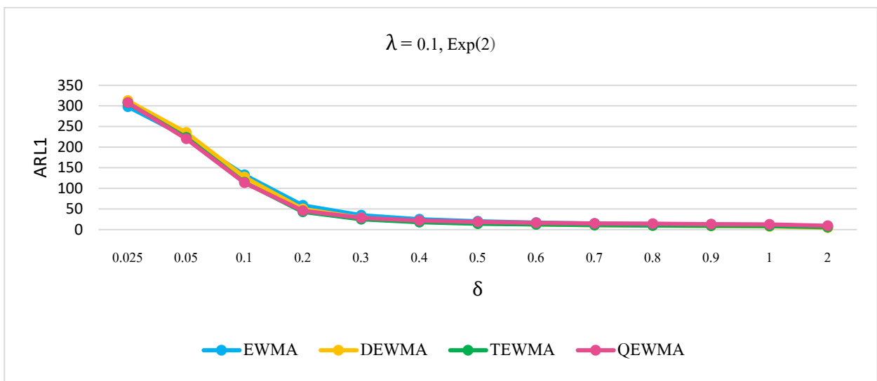
รูปที่:5 ค่า ARL_1 กรณี \lambda=0.10 ที่มีการแจกแจงแบบเลขชี้กำลัง \text{Exp}(2) ภายใต้อ ARL_0=370
