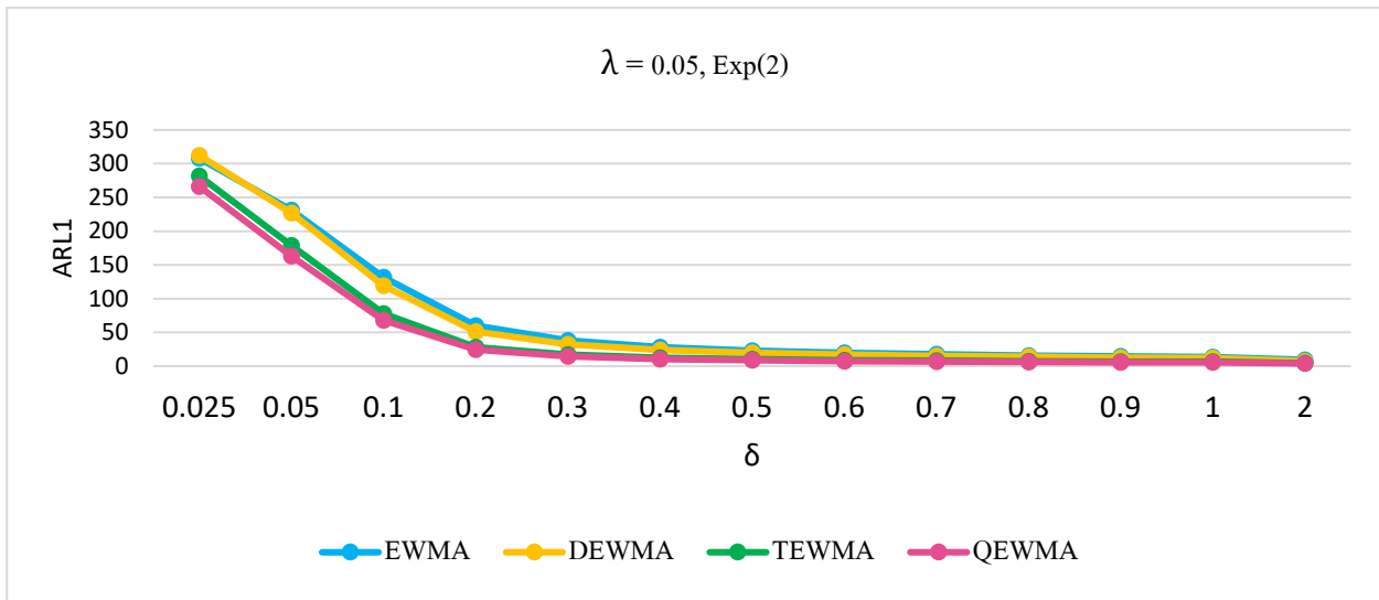
รูปที่: 4 ค่า ARL_1 กรณี \lambda=0.05 ที่มีการแจกแจงแบบเลขชี้กำลัง \text{Exp}(2) ภายใต้อ ARL_0=370
