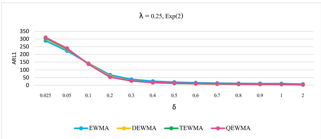
รูปที่: 6 ค่า ARL_1 กรณี \lambda=0.25 ที่มีการแจกแจงแบบเลขชี้กำลัง \text{Exp}(2) ภายใต้อ ARL_0=370
