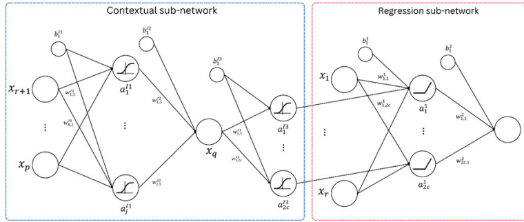
รูปที่ 1: โครงสร้างของโครงข่ายประสาทเทียมเชิงบริบท (CtxtNN)
