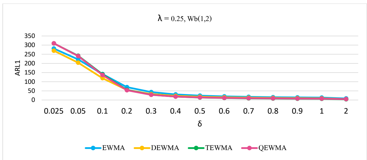
รูปที่: 9 ค่า ARL_1 กรณี \lambda=0.25 ที่มีการแจกแจงไวบูล Wb(1,2) ภายใต้ ARL_0=370
