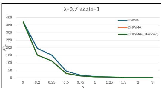
ภาพที่ 5 : การเปรียบเทียบค่า ARL ของแผนภูมิควบคุมเมื่อข้อมูลเป็นการแจกแจงโลจิสติกส์ ที่ \lambda = 0.7 และพารามิเตอร์ เท่ากับ 1
