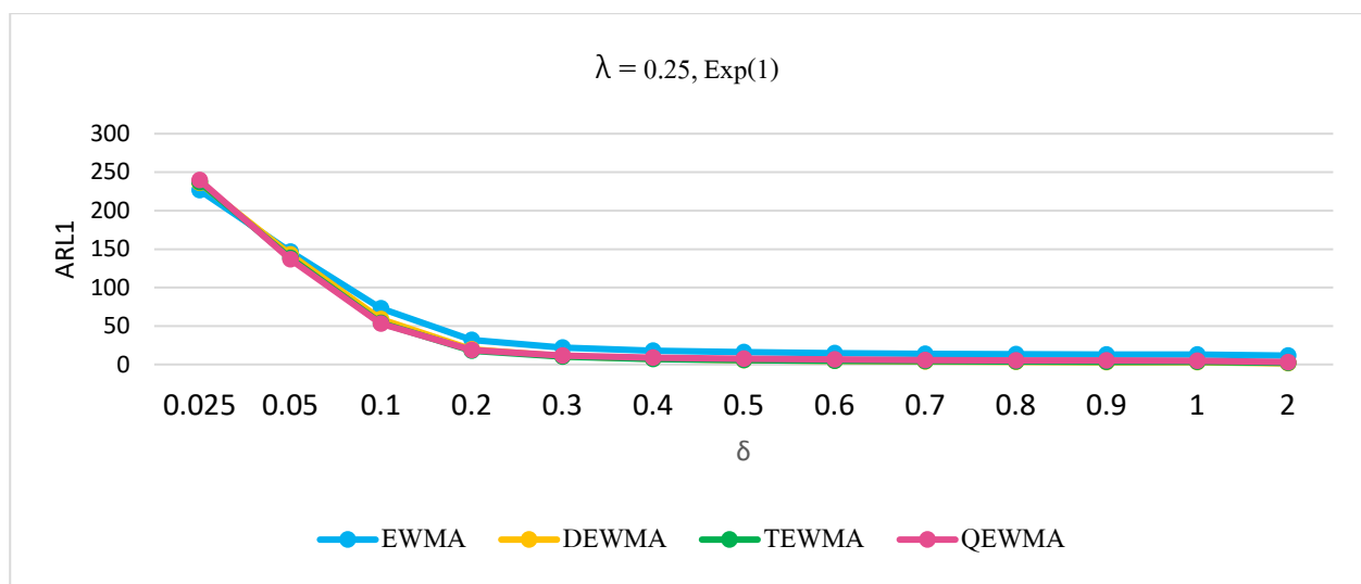
รูปที่: 3 ค่า ARL_1 กรณี \lambda=0.25 ที่มีการแจกแจงแบบเลขชี้กำลัง \text{Exp}(1) ภายใต้ ARL_0=370
