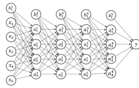
7(b) FNN-Small
