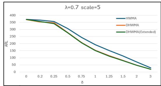
ภาพที่ 6: การเปรียบเทียบค่า ARL ของแผนภูมิควบคุมเมื่อข้อมูลเป็นการแจกแจงโลจิสติกส์ ที่ \lambda = 0.7 และพารามิเตอร์ เท่ากับ 5
