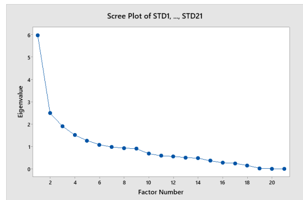
ภาพที่ 2: กราฟ Scree Plot
