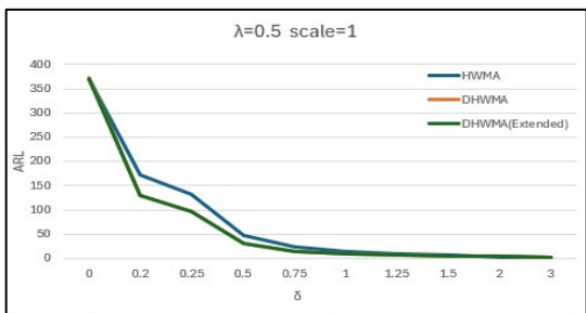
ภาพที่ 3: การเปรียบเทียบค่า ARL ของแผนภูมิควบคุมเมื่อข้อมูลเป็นการแจกแจงโลจิสติกส์ ที่ \lambda = 0.5 และพารามิเตอร์ เท่ากับ 1
