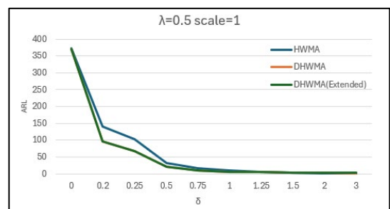
ภาพที่ 9: การเปรียบเทียบค่า ARL ของแผนภูมิควบคุมเมื่อข้อมูลเป็นการแจกแจงลาปลาซ ที่ \lambda = 0.5 และพารามิเตอร์ เท่ากับ 1
