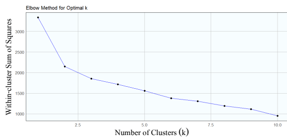
ภาพที่ 2: กราฟ Elbow Method สำหรับการกำหนดจำนวนกลุ่มที่เหมาะสมของข้อมูลชุดที่ 1
