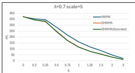
ภาพที่ 12: การเปรียบเทียบค่า ARL ของแผนภูมิควบคุมเมื่อข้อมูลเป็นการแจกแจงลาปลาซ ที่ \lambda = 0.7 และ พารามิเตอร์เท่ากับ 5
