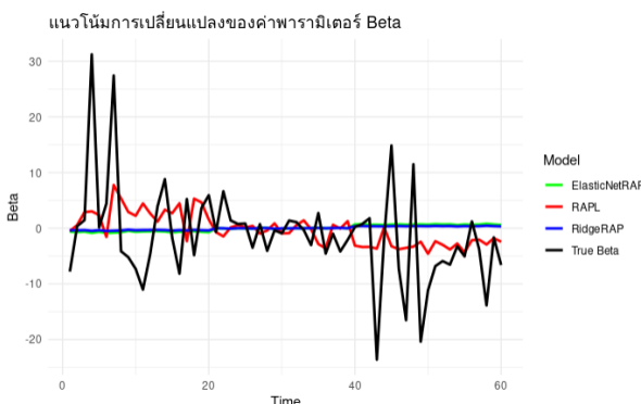
ภาพที่ 1: แนวโน้มการเปลี่ยนแปลงของค่าพารามิเตอร์สัมประสิทธิ์ภายใต้รูปแบบข้อมูลที่มีการเปลี่ยนแปลงต่ำ
