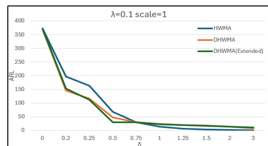
ภาพที่ 1: การเปรียบเทียบค่า ARL ของแผนภูมิควบคุมเมื่อข้อมูลเป็นการแจกแจงโลจิสติกส์ ที่ \lambda = 0.1 และพารามิเตอร์ เท่ากับ 1
