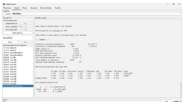
ภาพที่ 4: ผลแบบจำลอง K-Nearest Neighbours (KNN)
