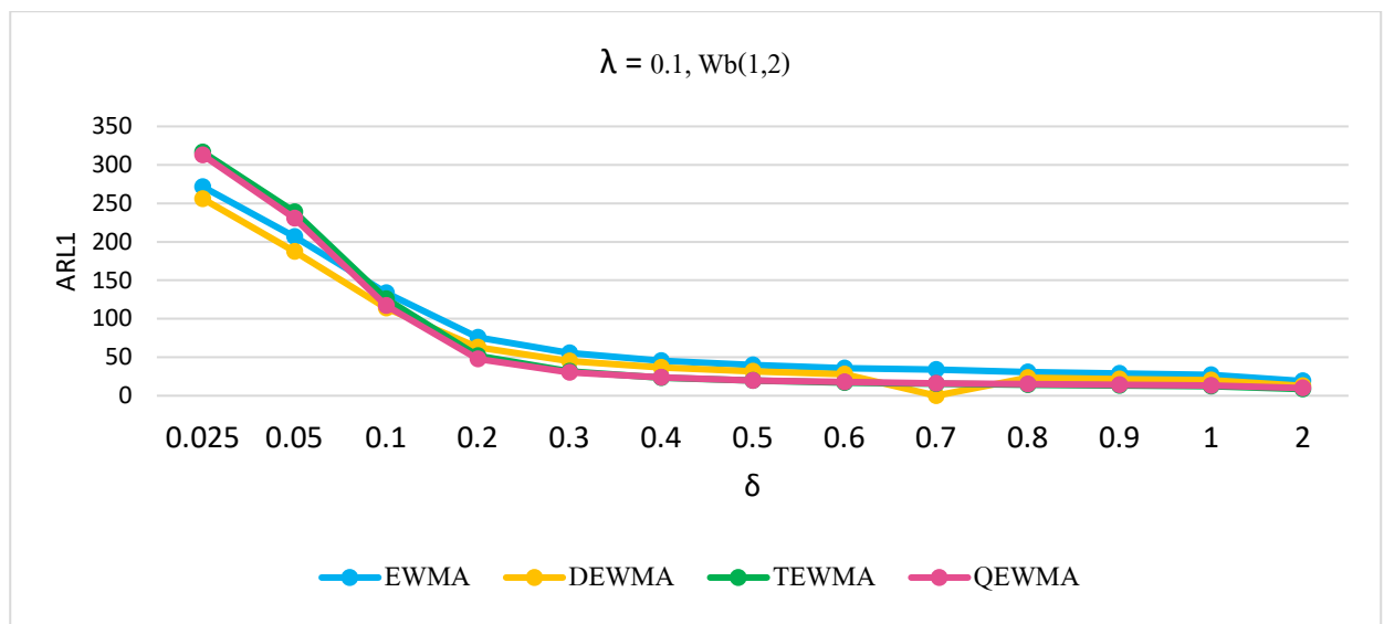
รูปที่: 8 ค่า ARL_1 กรณี \lambda=0.10 ที่มีการแจกแจงไวบูล Wb(1,2) ภายใต้ ARL_0=370
